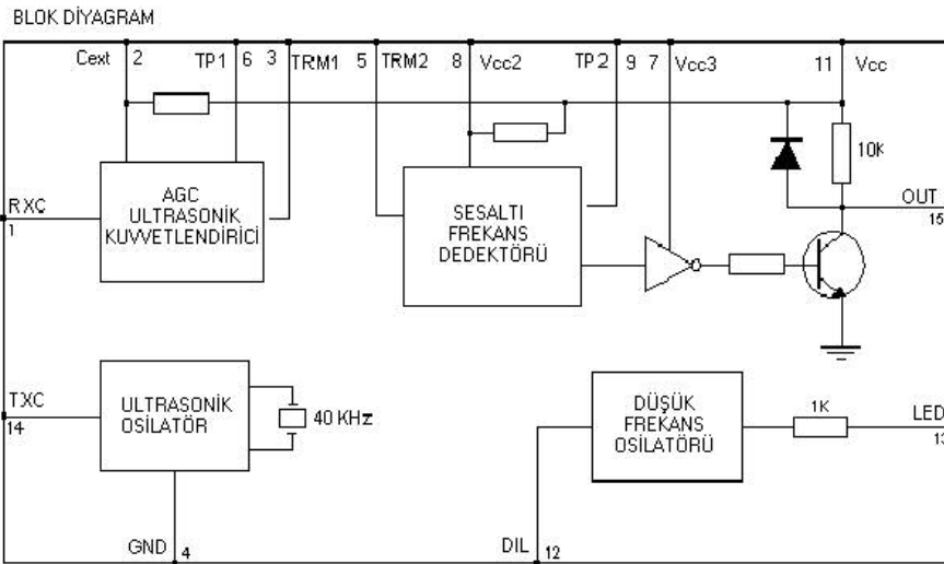
Şekil 3 Modülün blok diyagramı ve bağlantı uçları
