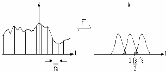
Şekil 5.2 Ayrık Fourier Dönüşümünde örnekleme frekansı çok düşük seçilirse frekans spektrumunda üstüste gelmeler olur.
